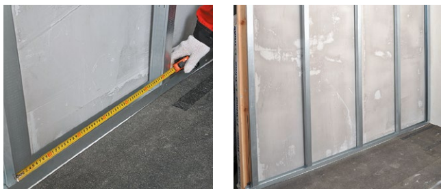
Рис. 6.10. Установка направляющего и стоечного профилей
