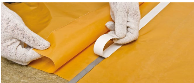
Рис. 5.3. Монтаж и проклейка нахлестов пароизоляционной пленки
