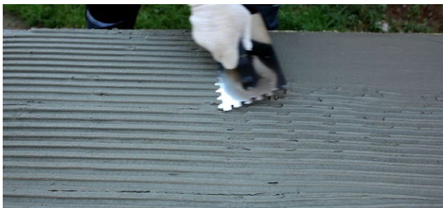
Рис. 7.28. Нанесение клеевого состава на плиту сплошным методом приклейки
