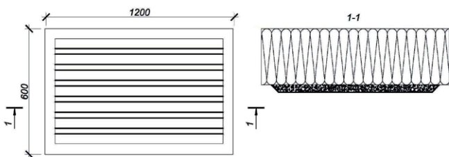
Рис. 7.29. Схема нанесения клея сплошным методом
