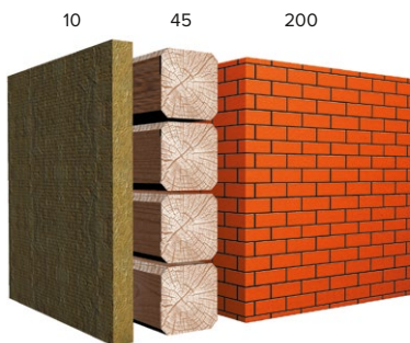
Рис. 1.1. Сравнение материалов при одинаковой теплосберегающей способности
